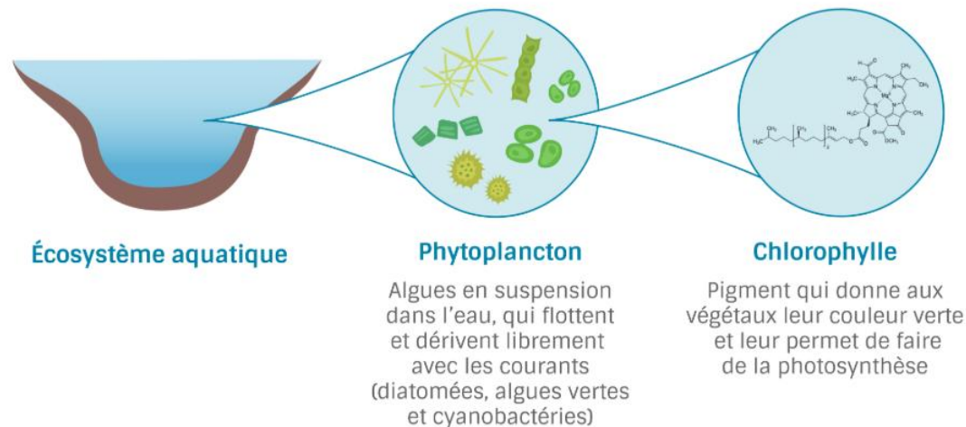
Schéma : L'origine de la chlorophylle mesurée dans l'eau d'un lac
